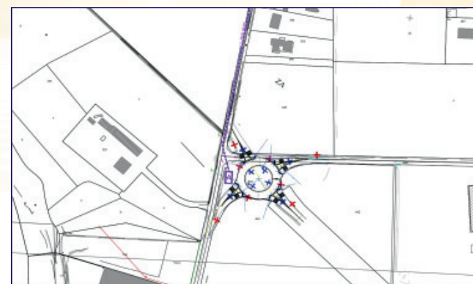
Rabattement des effluents de Larche plan d'implantation de la station de pompage à Laumeuil
